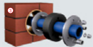
Photo : passe mur DN 100
