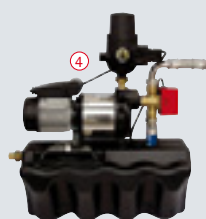
Coffret d'alimentation sur console avec pompe Superinox 15/4
